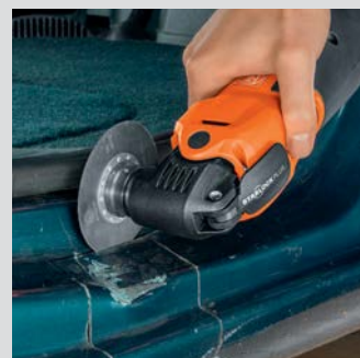
Pilování bez deformace, čisté řezné hrany, tenké linie řezu – výhoda u karosářských prací.
