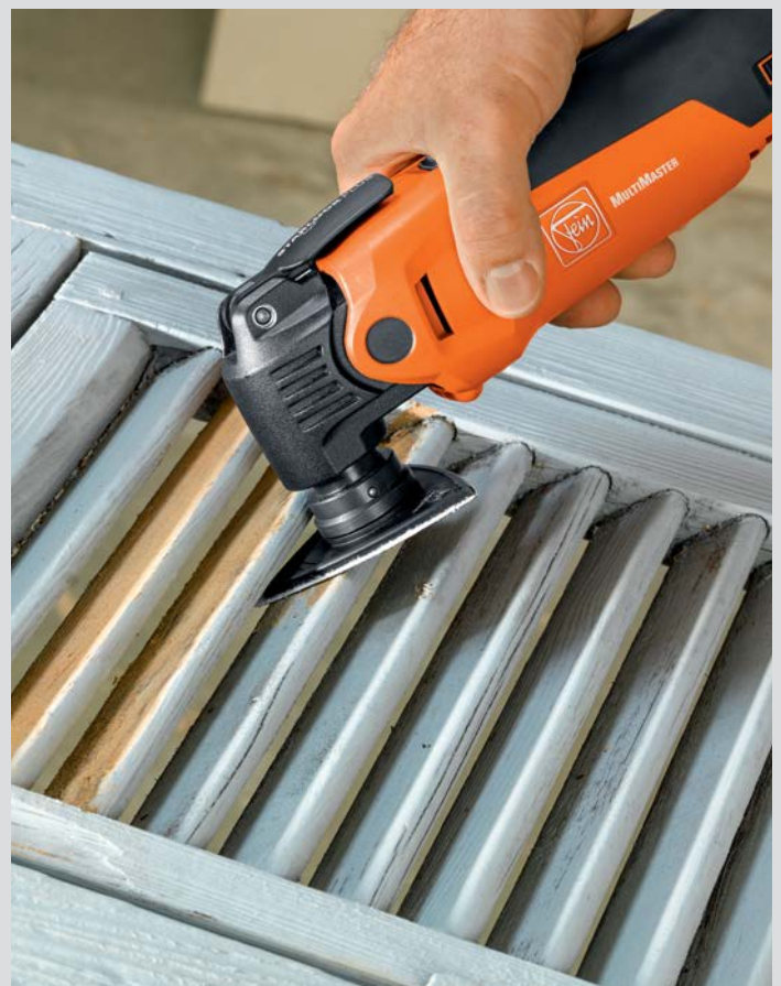
Plochá brusná deska pro úzké meziprostory.
