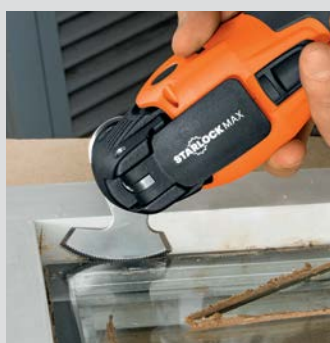
Oddělování izolačních skel uložených v tmelovém lůžku.
